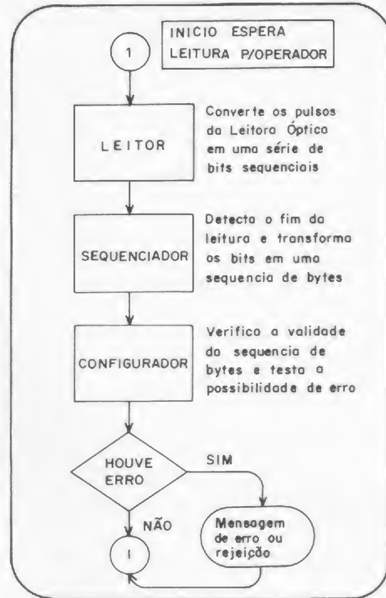
Figura 4 — Esquema simplificado do software de decodificação dos códigos de barras.
